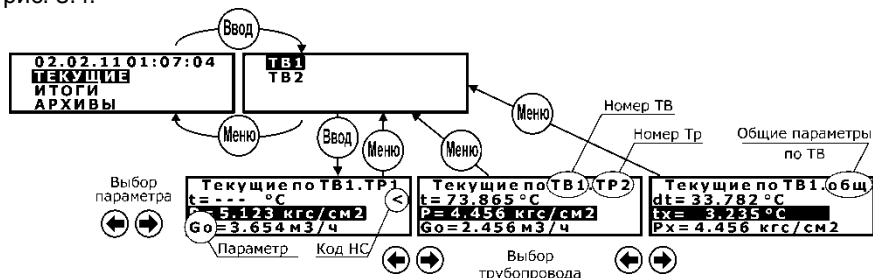
Рис. 3.3 – Пример просмотра текущих параметров
