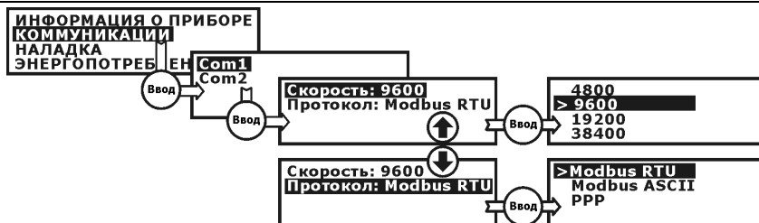
Рис. 3.10 – Настройка Com-портов
