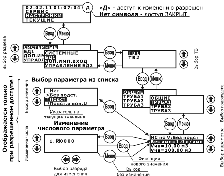
Рис. 3.1 – Пример просмотра значения параметра настройки
