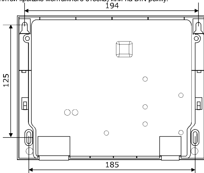
Рис. 4.1 – Схема крепления корпуса MBT-2М нк
