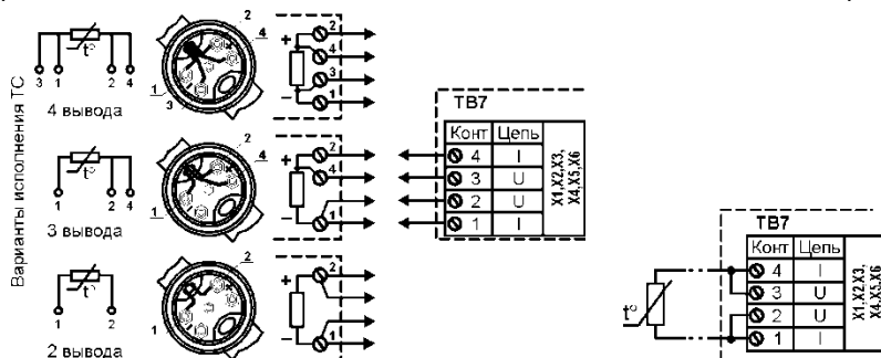
Рис. 4.2 - Варианты подключения ТС
