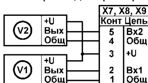
Рис. 4.3 Подключение УЗ счетчиков с питанием от тепловычислителя
